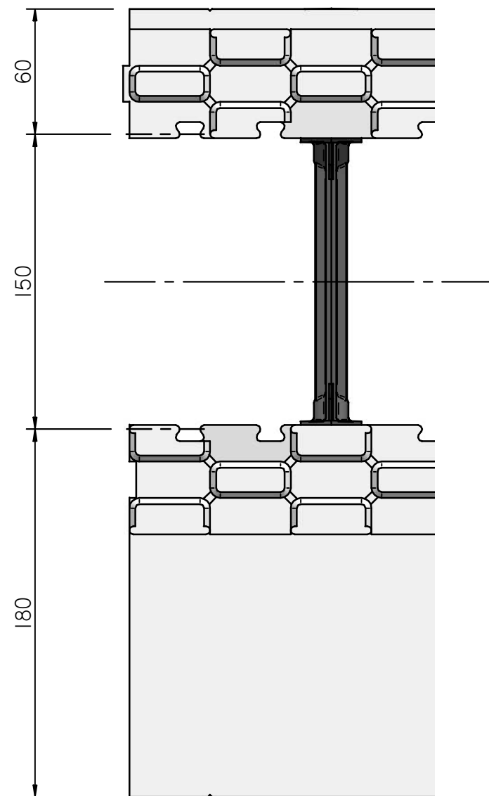
VISTA IN PIANTA DETTAGLIO
