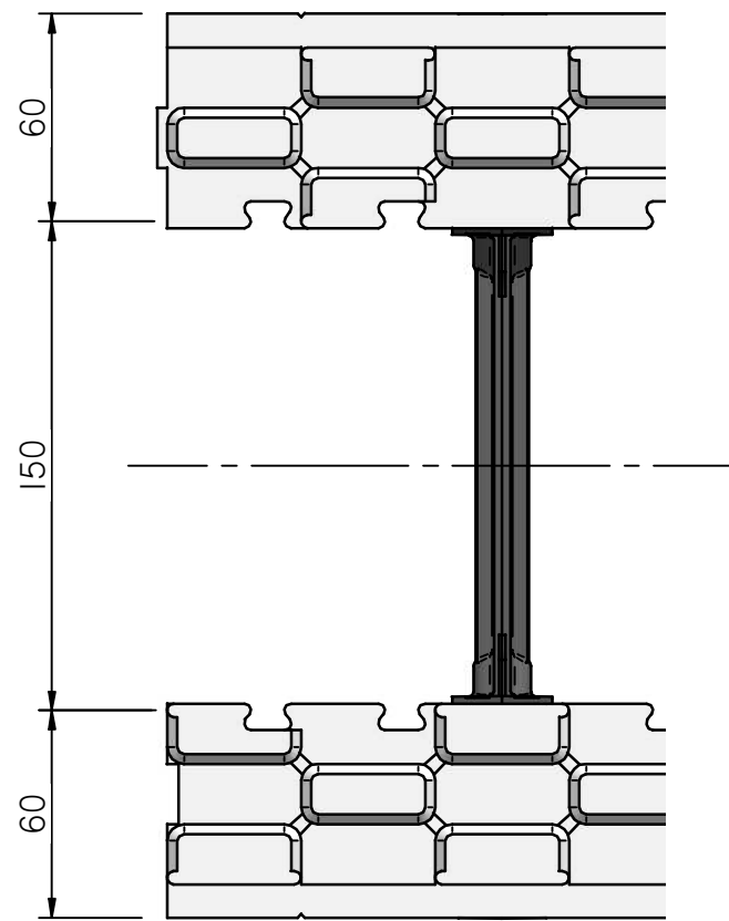
VISTA IN PIANTA DETTAGLIO
